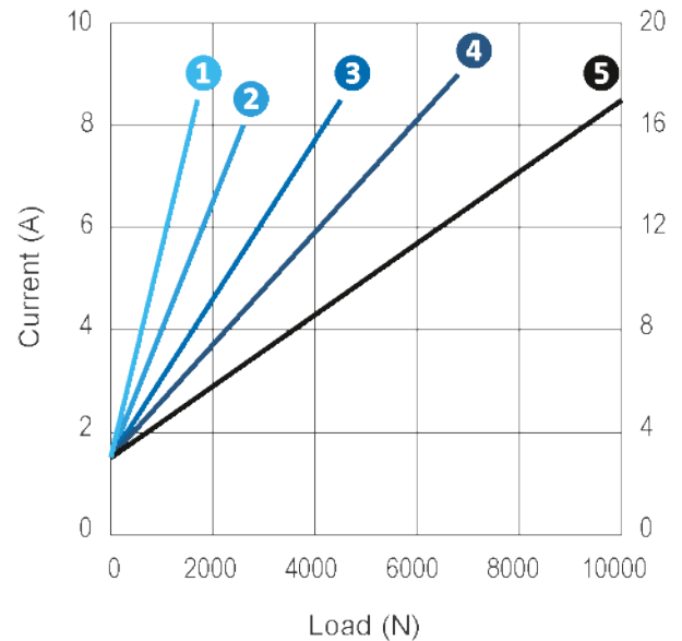
24V DC
