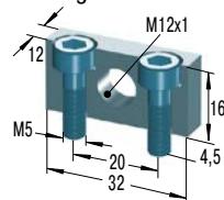
MB12SC2 Montageblok
