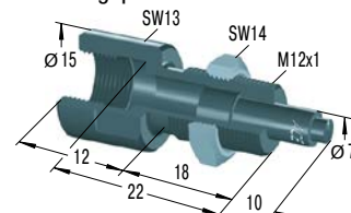
BV12SC Geleidingspen
