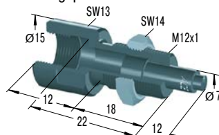
BV12 Geleidingspen
