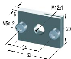
RF12 Rechthoekflens
