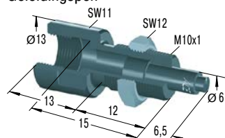
BV10 Geleidingspen
