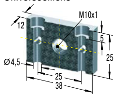
UM10 Universeelflens
